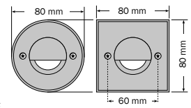
Alu eloxiert und weiß beschichtet anodised aluminum and coated white aluminium éloxé et laqué blanc
