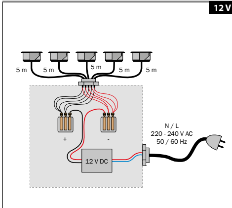
Akzentlichtpunkt 5er Set Anschlussplan outdoor Accent light point set of 5 wiring diagram outdoor Plan de câblage de lot de 5 pour l'extérieur
